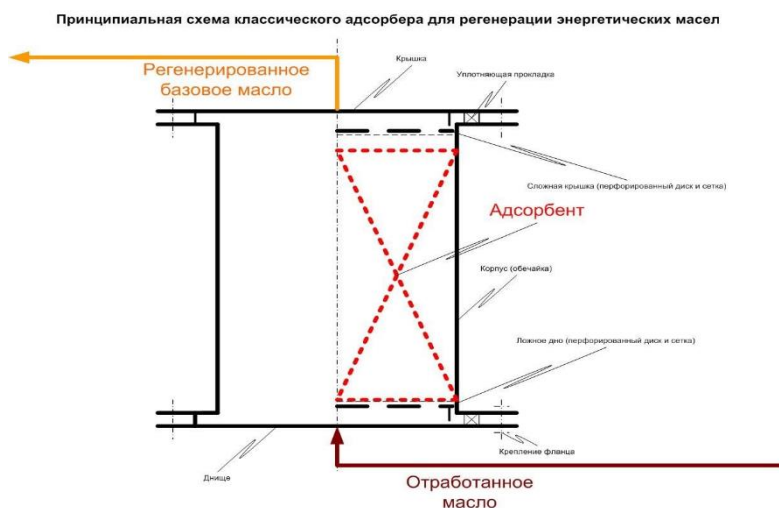
Рисунок № 1. Схема адсорбера
