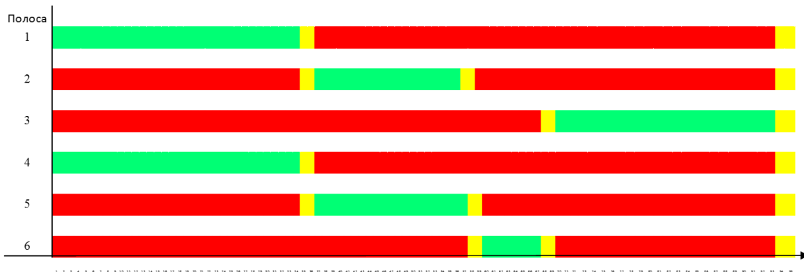
Рис. 5. Фазы работы светофоров на перекрестке ул. Холмогорова и ул. Пушкинская
