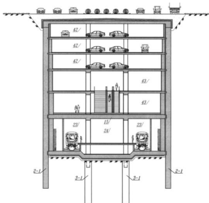
Рисунок 1 –Макет строительства станции метрополитена
