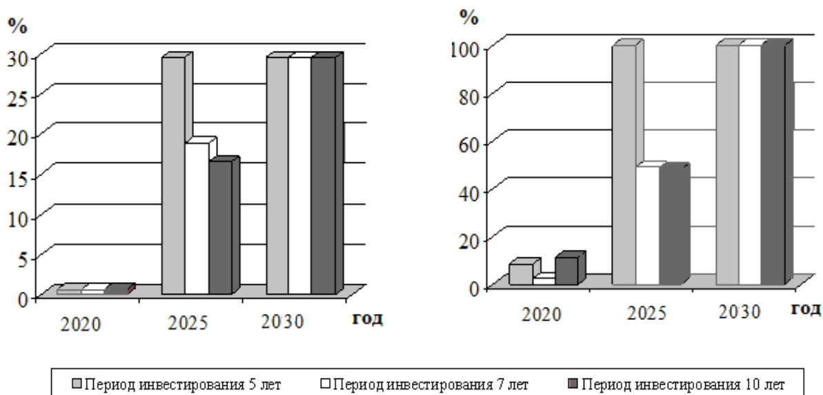
Рис. 4, а – Динамика индикатора “Процент местных видов ТЭР” при различных периодах инвестирования
