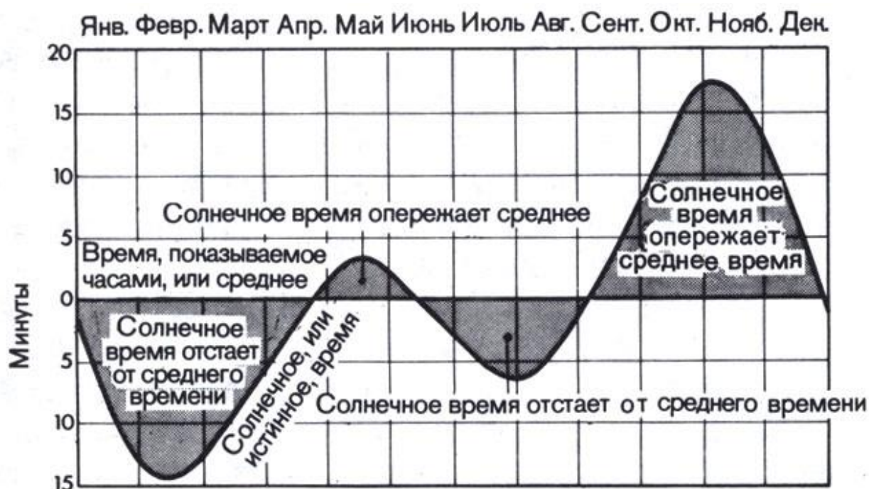
Рис.1 График УВ
